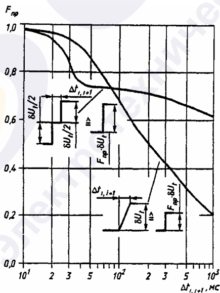
Рисунок В.1. Коэффициент приведения F_{пр} для периодических колебаний напряжения, имеющих двухступенчатую и пилообразную
