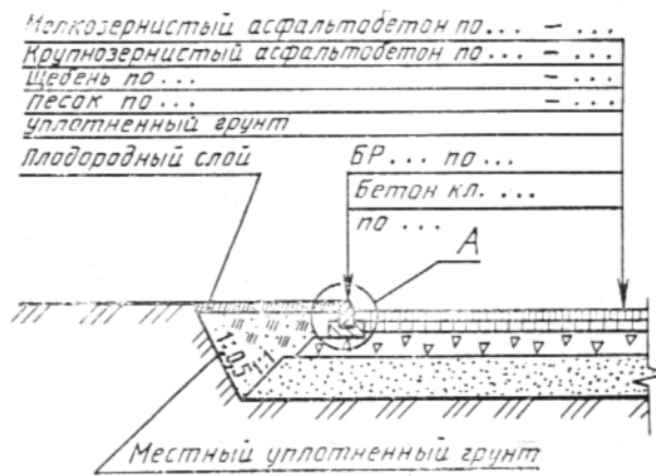
Тротуар (тип 2)
