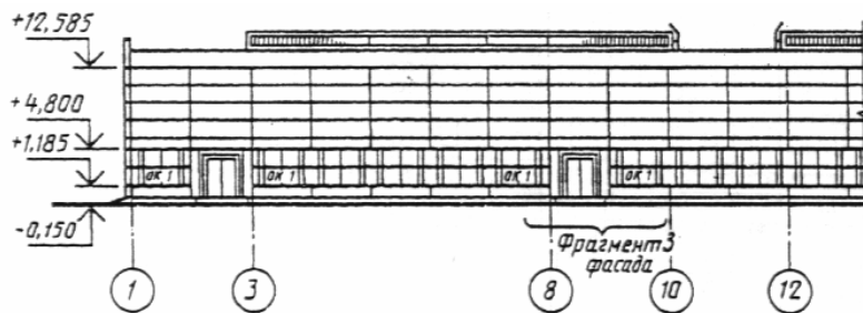
Фасад 1-22.
